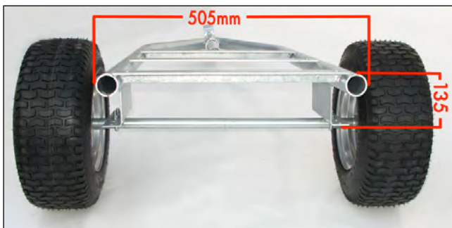
Anhängerchassis Rückansicht
